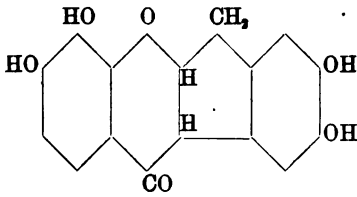
Hämatein
